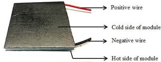
Fig. 3. Single TEG module.
