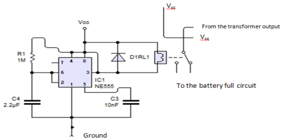
404 Fig.: 9 Delay circuit
