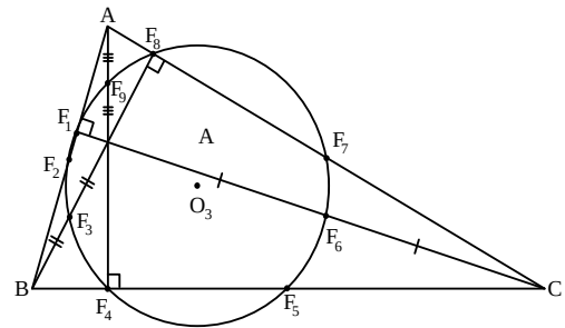
Fig. 1. The 9 point circle
