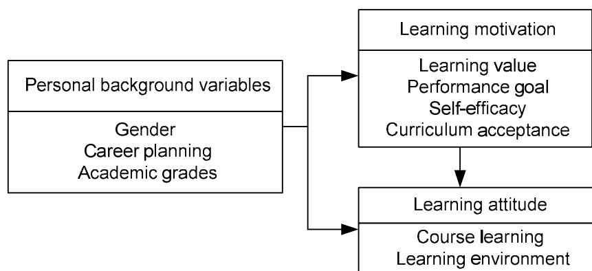
Figure1 : Framework
