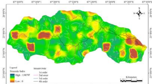
(H) Sinuosity Index
