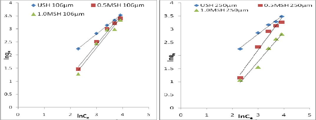
215 Fig. 6: Freundlich Isotherm for \text{Ni}^{2+} 106 \mu\text{m} (a) 216 Freundlich Isotherm for \text{Ni}^{2+} 250 \mu\text{m} (b) 217
