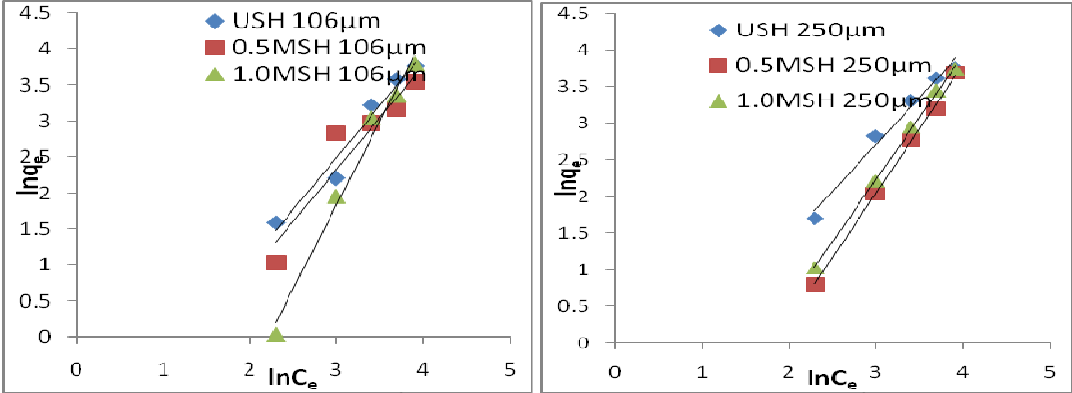
222 Fig. 8: Freundlich isotherm for \text{Zn}^{2+} 106 \mu\text{m} (a) 223 Freundlich isotherm for \text{Zn}^{2+} 250 \mu\text{m} (b) 224
